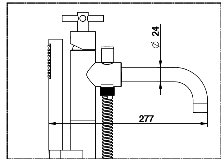
DETTAGLIO A
