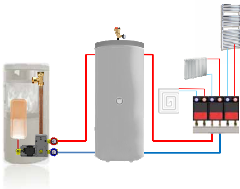
Impianto di riscaldamento, accumulo e generatore a biomassa con kit.
