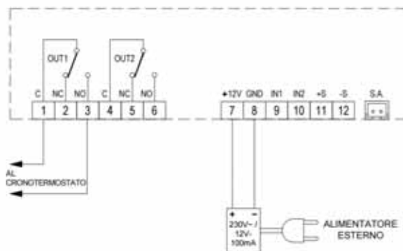
Esempio di collegamento ad un cronotermostato.
