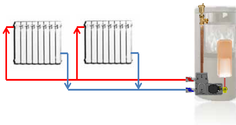
Impianto di riscaldamento e generatore a biomassa con kit.
