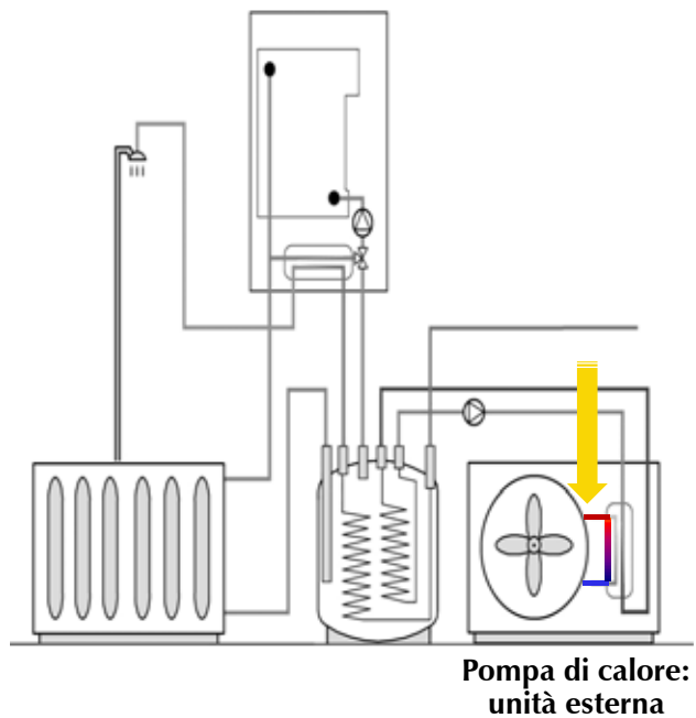
FIGURA 1 - FUNZIONAMENTO PDC: CIRCUITO CHIUSO;
