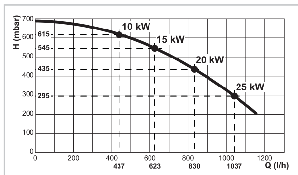
Prevalenze residue pompa caldaia a bordo Calenta 15s-25s-28c
