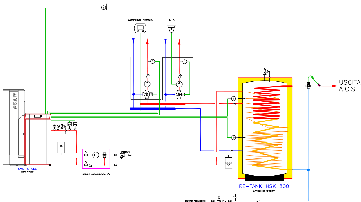
SCHEMA 2: SISTEMA CON CALDAIA A PELLET PER RISCALDAMENTO E PRODUZIONE SEMI ISTANTANEA DI A.C.S.
