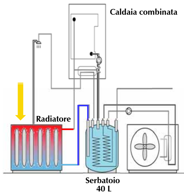
FIGURA 3 - PRERISCALDO RISCALDAMENTO;
