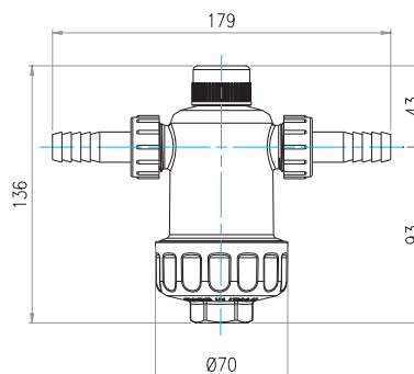
Configurazione 2: Raccordi portagomma dritti
