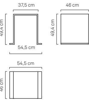
TAVOLINO COLLEGAMENTO / CONNECTION TABLE
