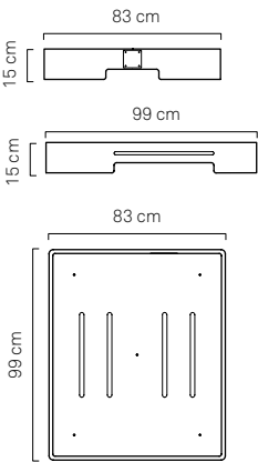
BASAMENTO POLTRONA / ARMCHAIR PLEXI BASE
