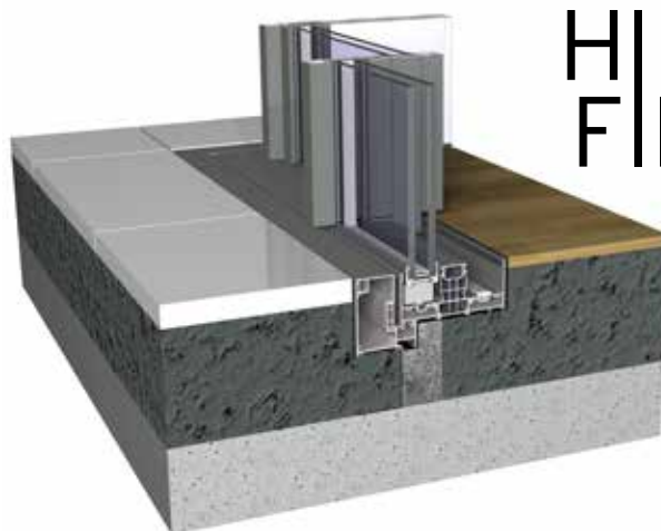
Sistema scorrevole panoramico Hi-Finity - sezione 3D
