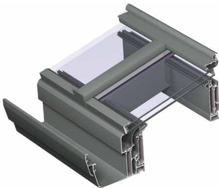
Sistema per verande e coperture tetti CR 120
